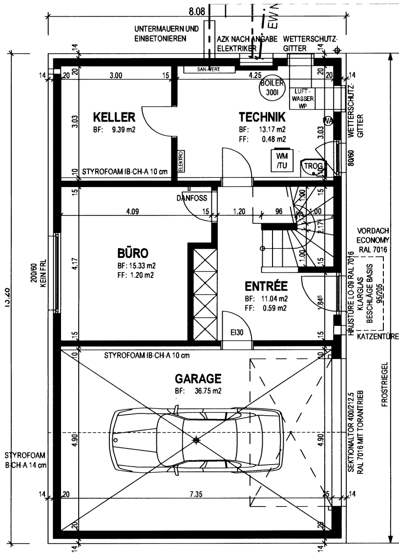
GRUNDRISS KELLERGESCHOSS
