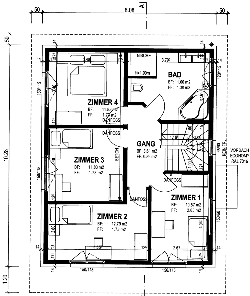
GRUNDRISS DACHGESCHOSS
